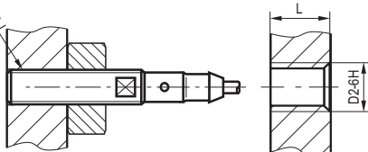
Схема монтажа
